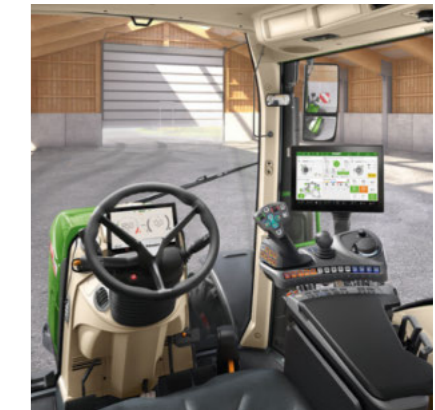
Profi+ Setting 1 - Krydsgreb - Et lineært modul (vippepar) til betjening af hydrauliske ventiler - 12"-terminal
