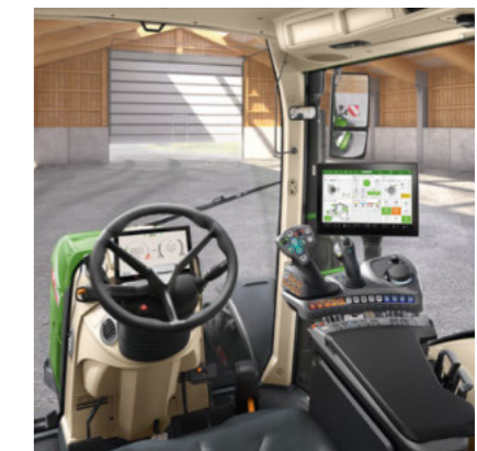
Profi+ Setting 2 - 3L-joystick - Et lineært modul (vippepar) til betjening af hydrauliske ventiler - 12"-terminal
