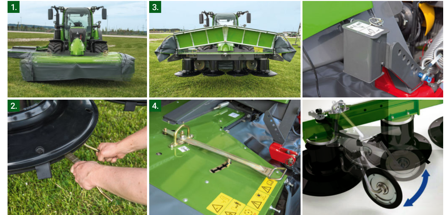
Pendelslag +/- 5°
